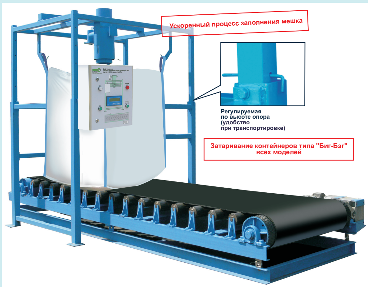
Надежный мотор-редуктор фирмы Bonfiglioli
